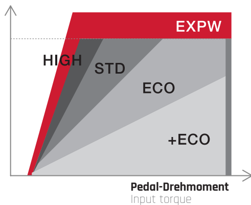
Motor-Drehmoment Motor torque
